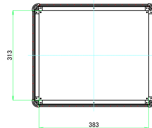
C-C ( 1 : 6.5 )
